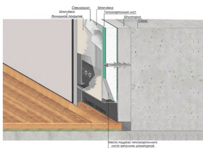
Примыкание к двери открытого монтажа
