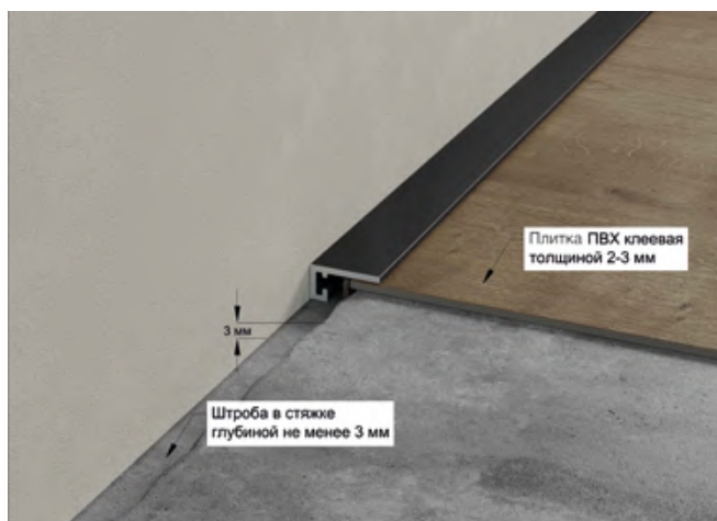
Решение с клеевой плиткой ПВХ
