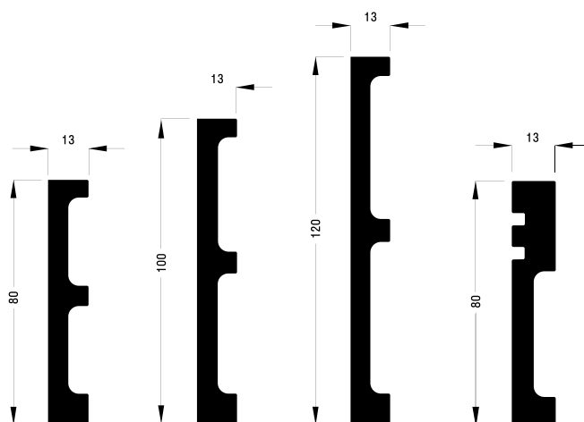
Декоративные вставки из водостойкого дюрополимера
