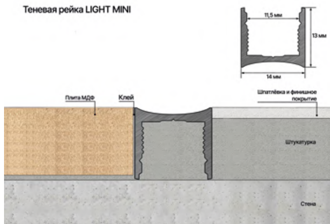
Заглушка к теневой рейке LIGHT MINI Вид сверху
