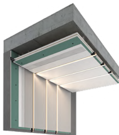
Рейка с заходом на потолок
