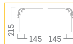
УЗЕЛ 66046RC (215*145 ММ)
